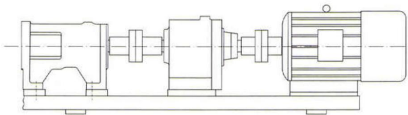
齿轮配合普通电机驱动
